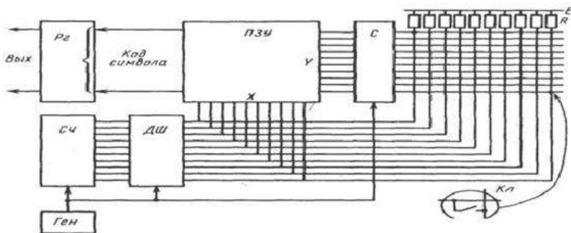
Рисунок 1 - Структурная схема контроллера.
