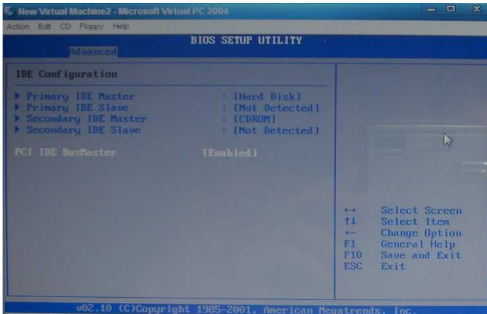
Рис. 6 Virtual Machine
