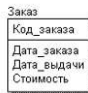
Рис. 2.9. Сущность Заказ
