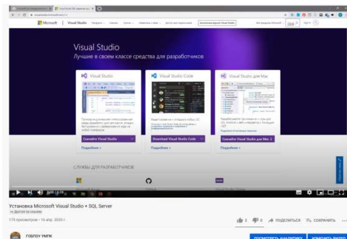
Рис.1 – Установка ПО
