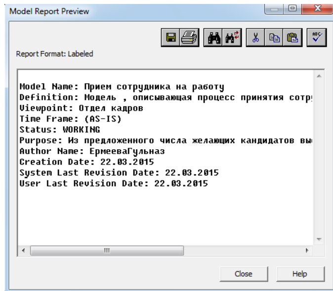
Рисунок 3 Отчет ModelReport
