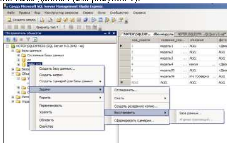
Рисунок 1 – Восстановление БД
