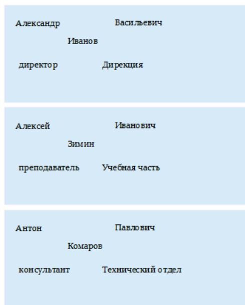
Рис. 8. Отчет «Представительский»
