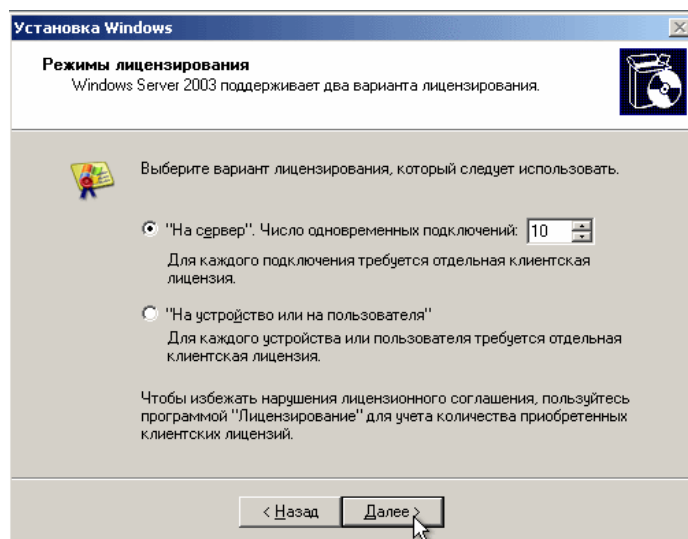
Рис.11. Вариант лицензирования.
